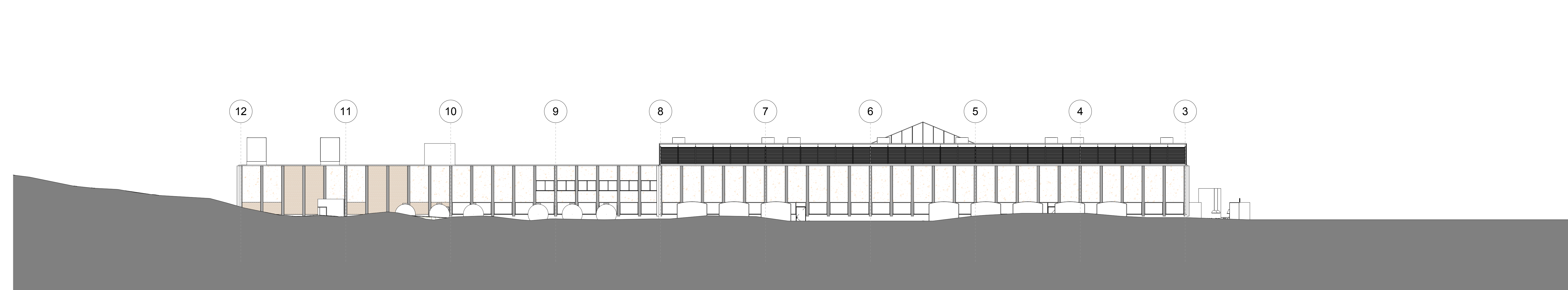
FASADE SYDØST
